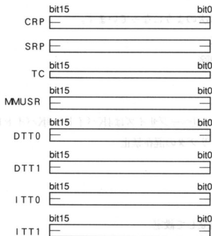
●図32……MC68040のMMU関連レジスタ
