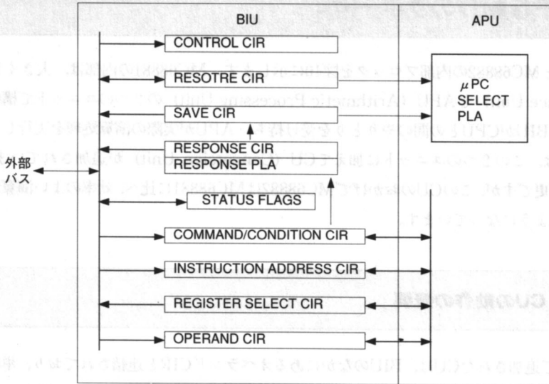
●図10……MC68881とMC68882の内部ブロック
