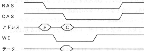
アーリーライト動作
