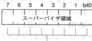
●図11……エリアセットポート(X68000/X68030共通)
