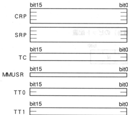
●図24……MC68030のMMU関連レジスタ
