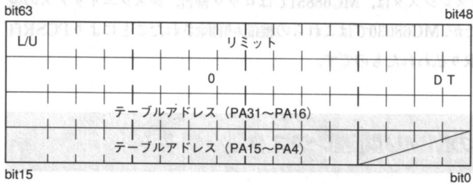
●図25……MC68030のSRP/CRP (ルート・インタレジスタ) のビット配置
