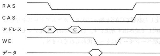
ディレイドライト動作
