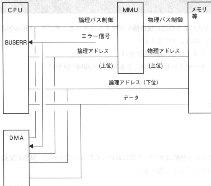
●図5 ……CPUとMMU、メモリの接続関係
