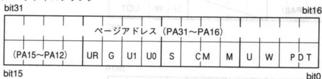
●図38……MC68040のページディスクリプタ
