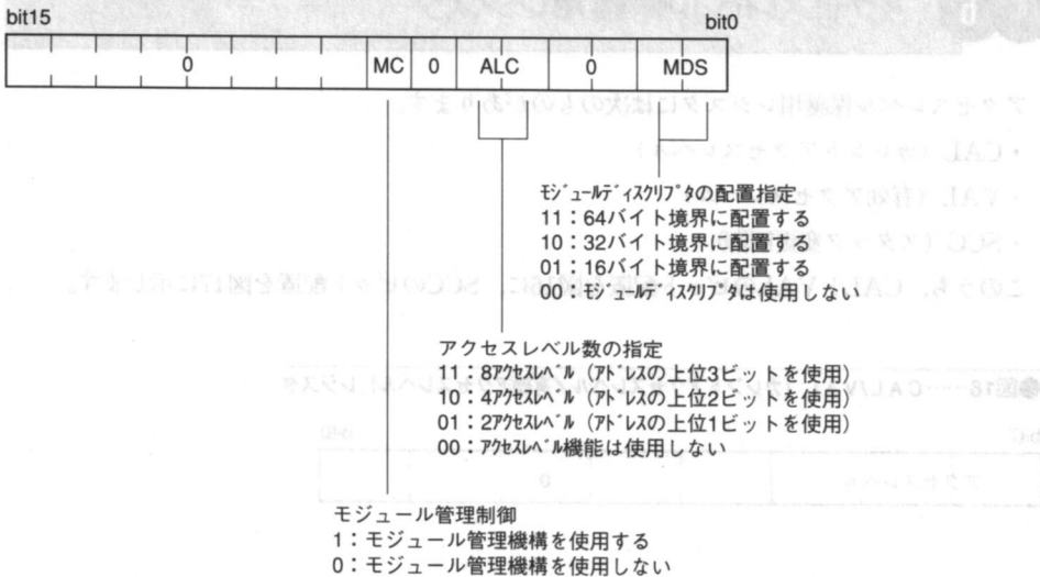
●図18……AC (アクセス制御) レジスタ
