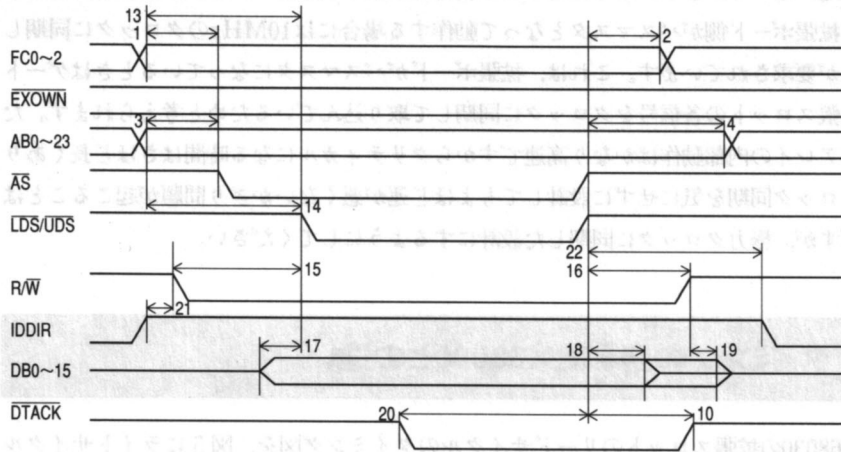
●図6……X68030拡張スロットタイミング値
