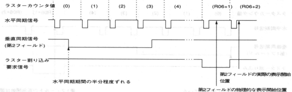
● 図11……第2フィールドの水平・垂直同期信号の波形とラスタカウンタの値
