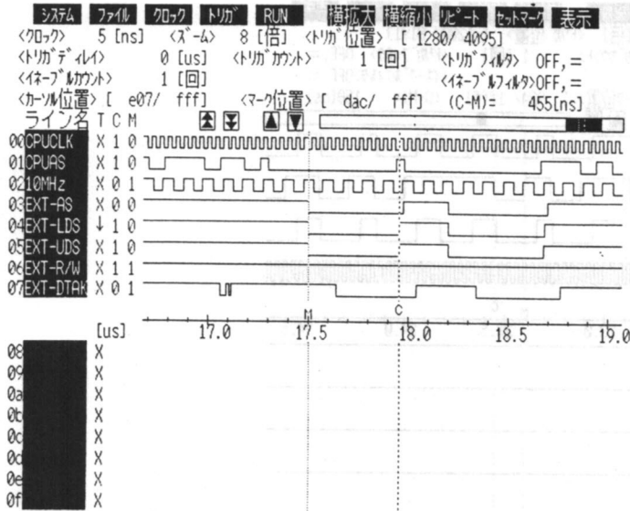
●図11……拡張スロットアクセス (カーソルはUDS/LDSの幅)
