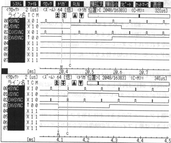
●図15……入力、本体ともインターレースのときの動作
