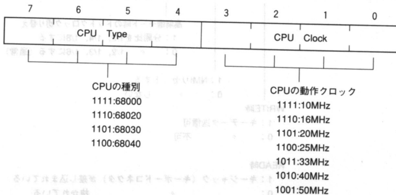
●図4 ……システムポート#6
