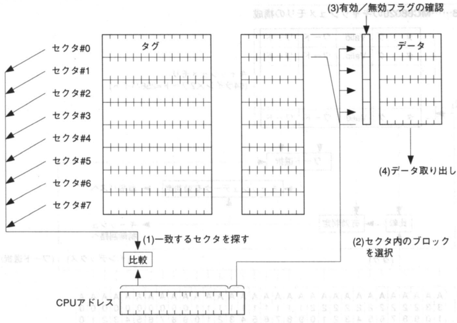
● 図17……セクタ方式
