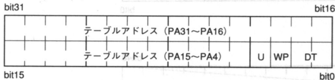
● 図29……MC68030のテーブルディスクリプタ
