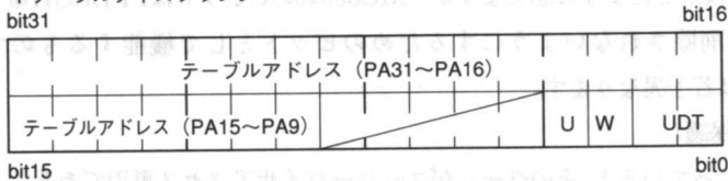
● 図37……MC68040のテーブルディスクリプタ
