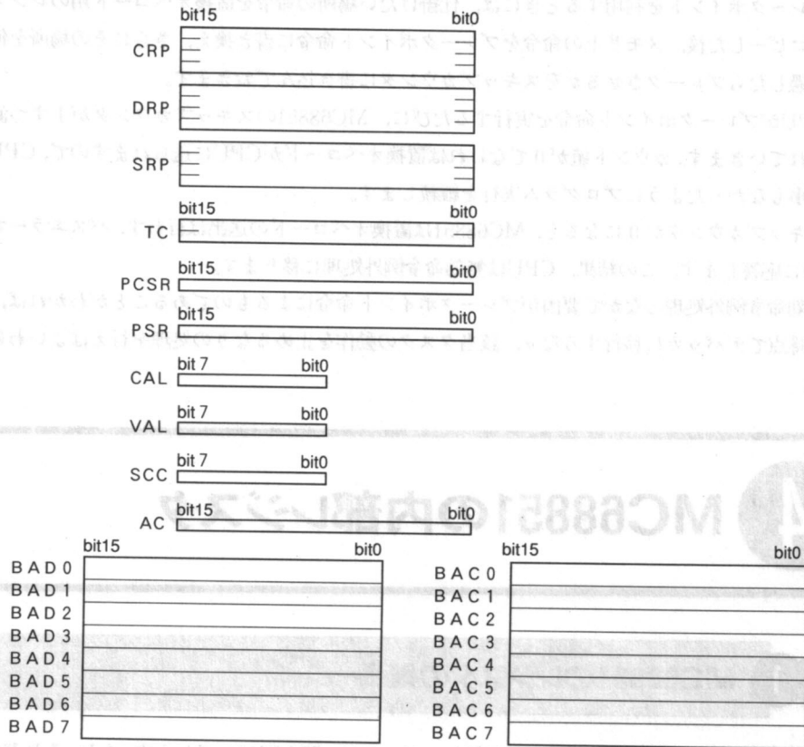
●図10……MC68851のレジスタ
