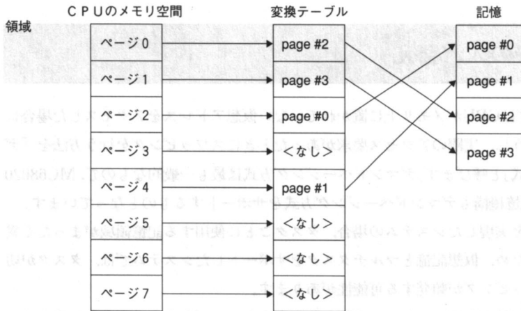
● 図 4 ……ページング方式
