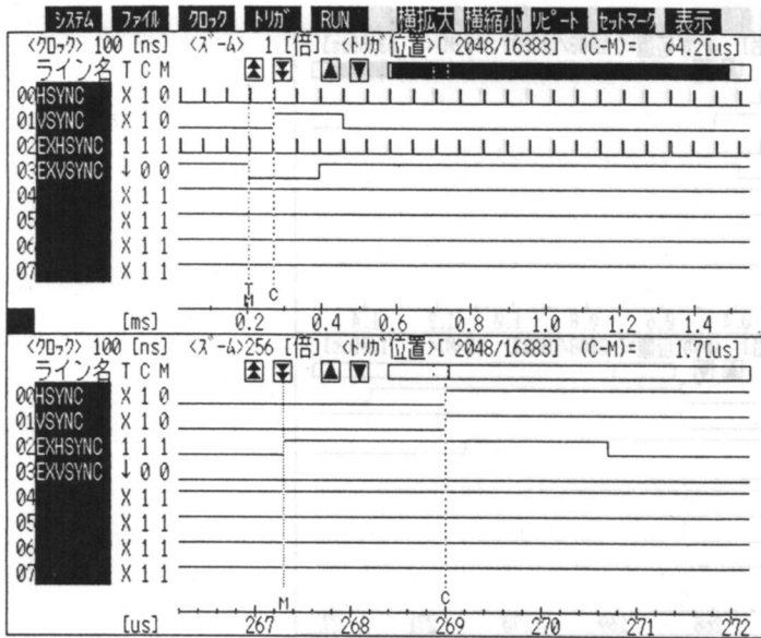
●図21……スーパーインポーズ動作時の波形 (R08に$40を設定)
