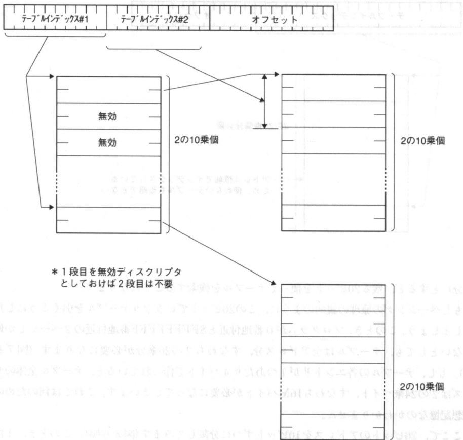
●図8 ……アドレスを2分割してテーブル量を節約
