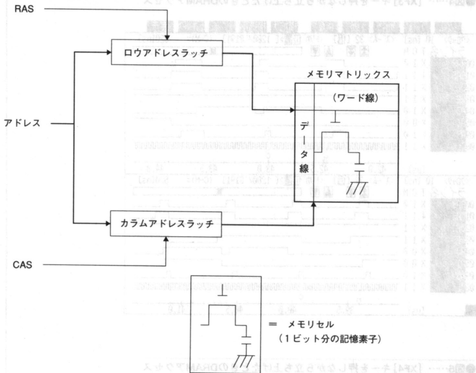
●図6……DRAMの内部構造
