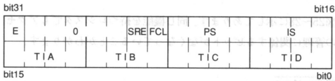
●図26……MC68030のTC (変換制御レジスタ) のビット配置
