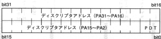
● 図39……MC68040の間接ディスクリプタ
