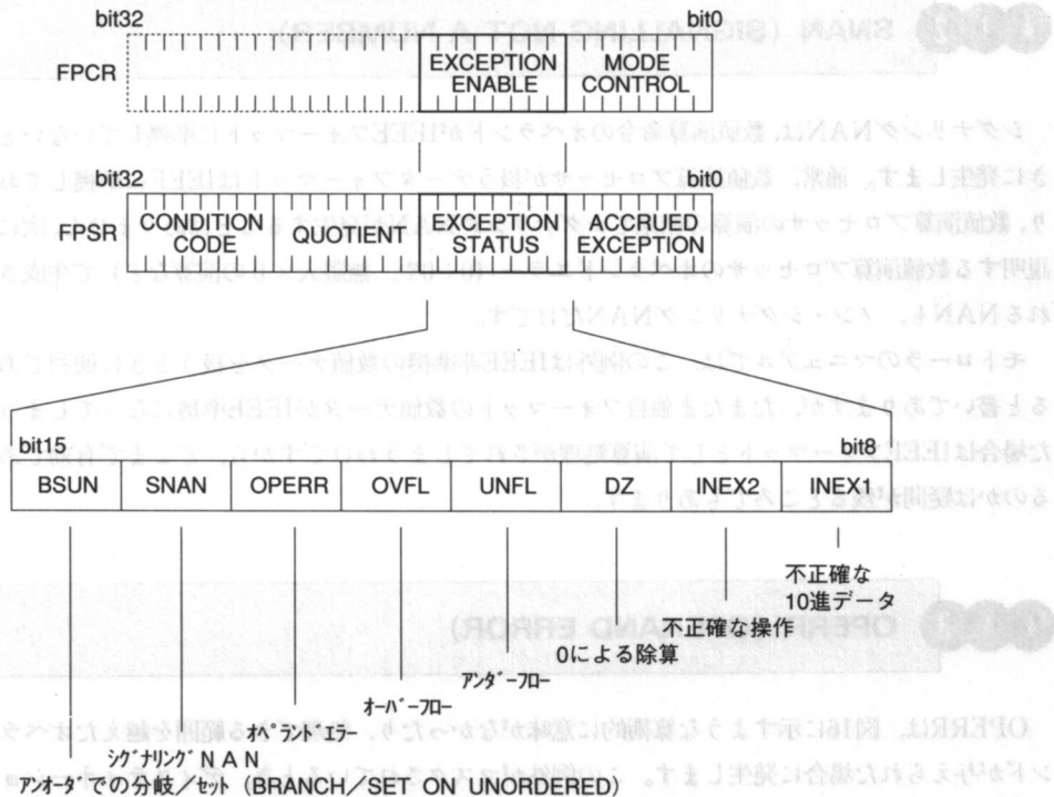
●図15……FPCR, FPSRの例外処理関連ビット
