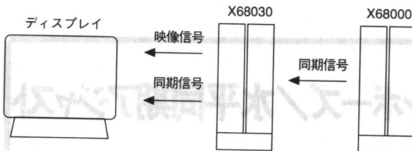
●図13……実験時の接続
