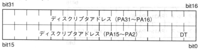
●図23……間接ディスクリプタ
