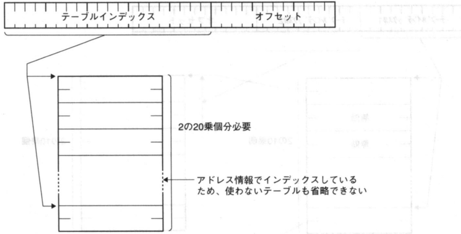
●図7……アドレスから直接テーブルを引く場合
