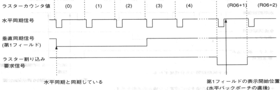
●図10……第1フィールドの水平・垂直同期信号の波形とラスタカウンタの値
