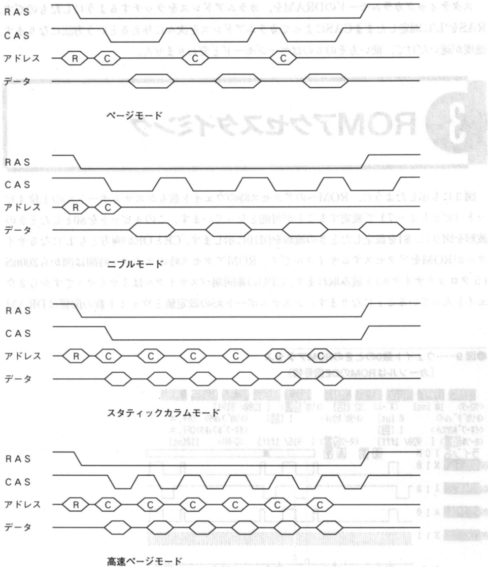
●図8……DRAMの高速アクセスモード
