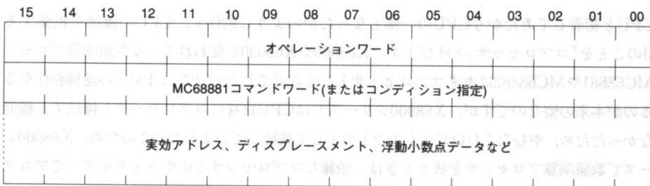
●図1……浮動小数点命令のフォーマット
