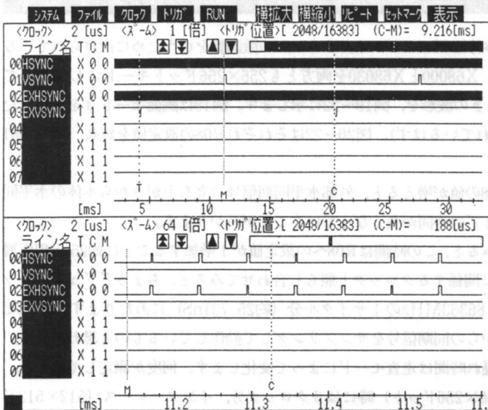
●図17……入力がノン・インターレース、本体はインターレースのときの動作
