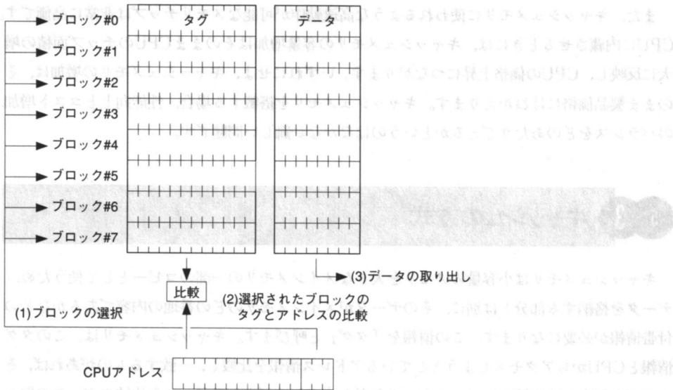
●図14……ダイレクトマップ方式
