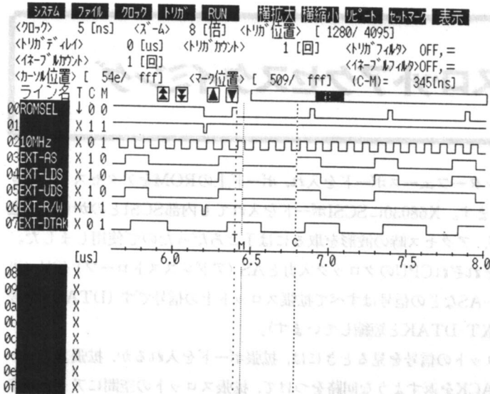
●図12……X68000での拡張スロットアクセス (カーソルはUDS/LDSの幅)
