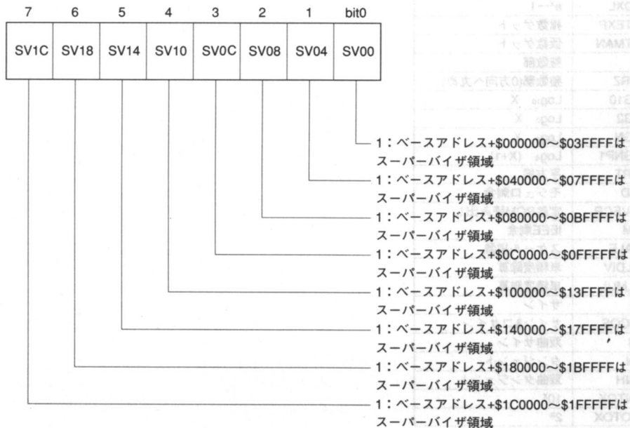
● 図12……拡張エリアセットレジスタ(X68030)
