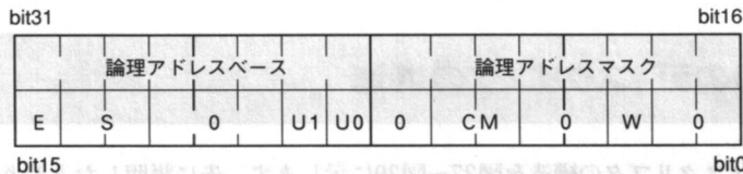
●図36……MC68040のDTT0/DTT1/ITT0/ITT1(透過変換レジスタ)のビット配置
