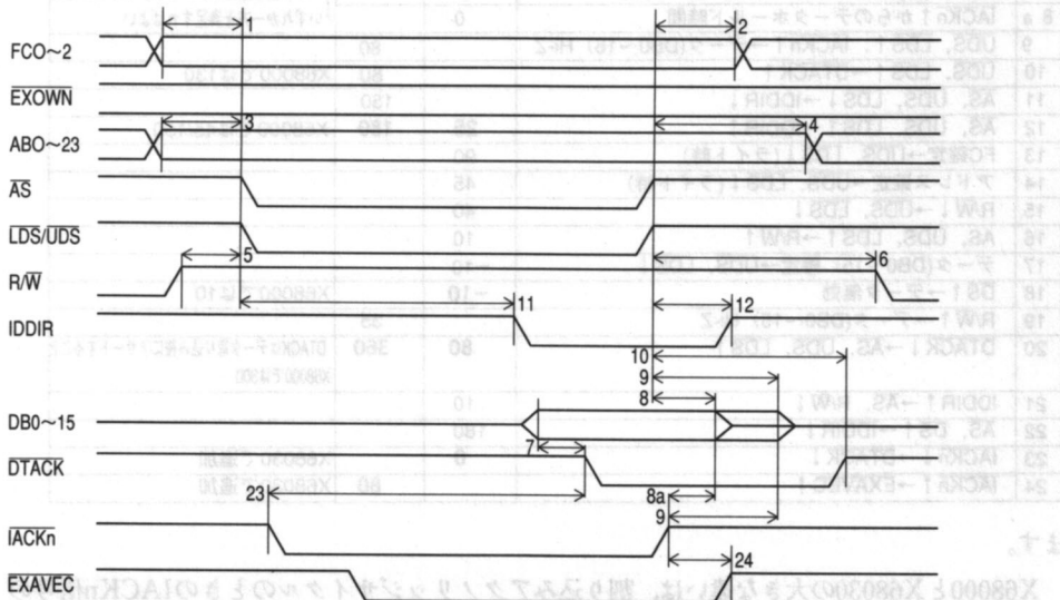
●図4……X68030拡張スロットリードサイクル
