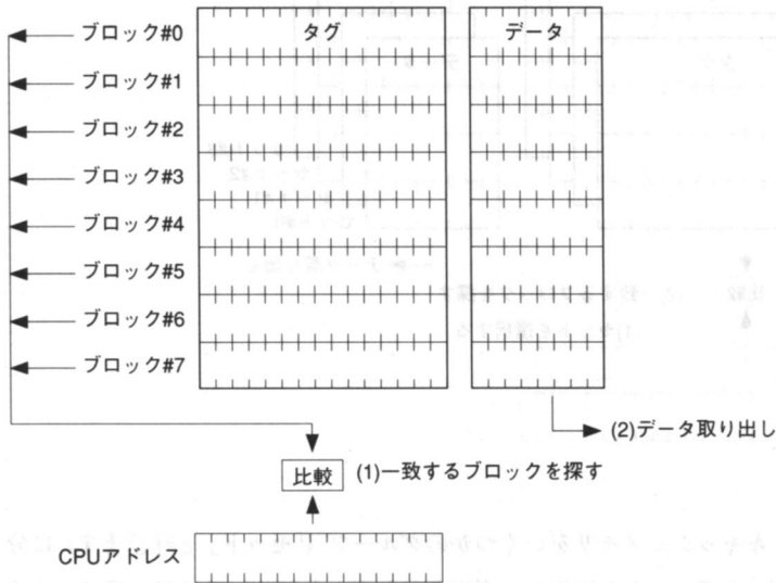
●図15……フルアソシエイティブ方式
