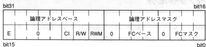
●図28……MC68030のTT0/TT1（透過変換レジスタ）のビット配置
