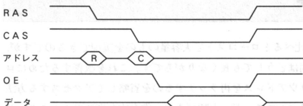
●図7……DRAMの基本アクセス
