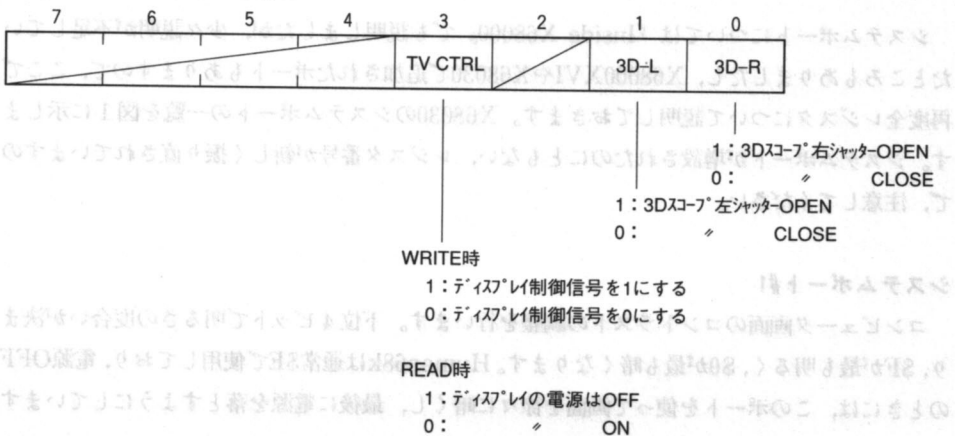
●図2……システムポート#2
