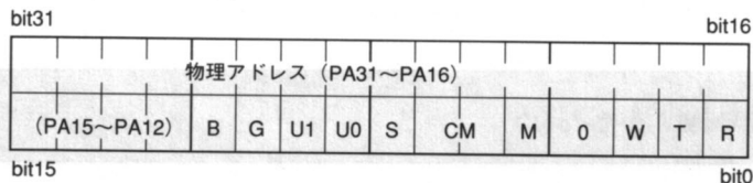
●図35……MC68040のMMUSRのビット配置
