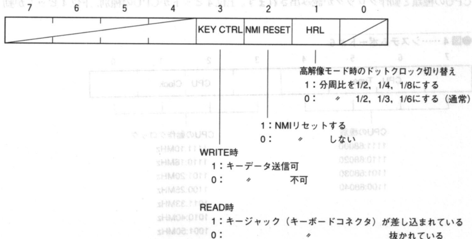
●図 3 ……システムポート #4
