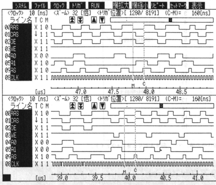
●図2……ウェイト数に$1を設定したときのアクセスタイミング (カーソルはDRAMのアクセスサイクル幅)
