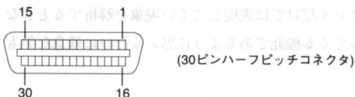
●図5……X68030イメージ入力端子ピン配置
